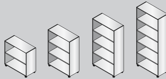
J9008G 90x39,6x83 h J9012G 90x39,6x121,4 h J9016G 90x39,6x159,8 h J9020G 90x39,6x201,4 h
